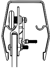
Perfil de aluminio satinado.
